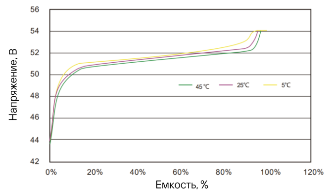
Зарядные характеристики 0.5C при различных температурах
