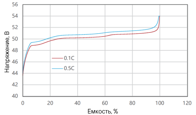
Зарядные характеристики при 25 °C
