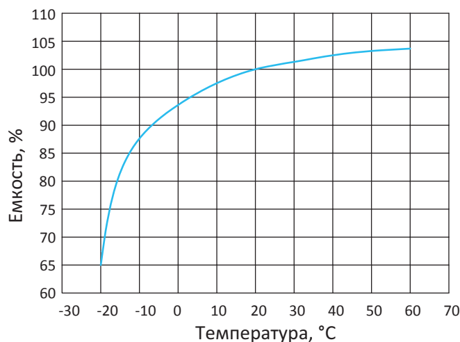
Отдаваемая емкость в зависимости от температуры
