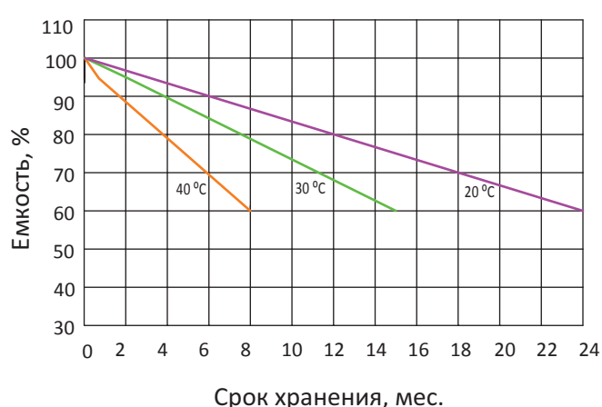
Саморазряд в зависимости от температуры хранения
