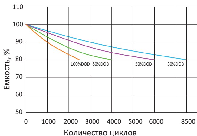
Количество циклов при разной глубине разряда
